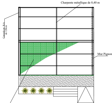
Plan de charpente
