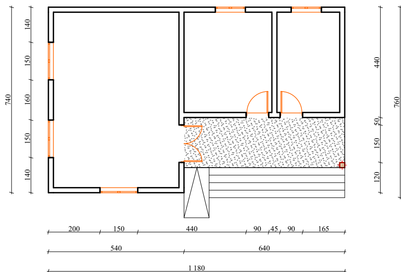
Plan coté
